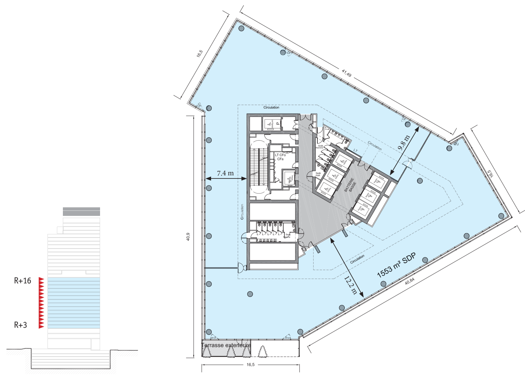
Plan type en batterie basse R+3 à R+16
