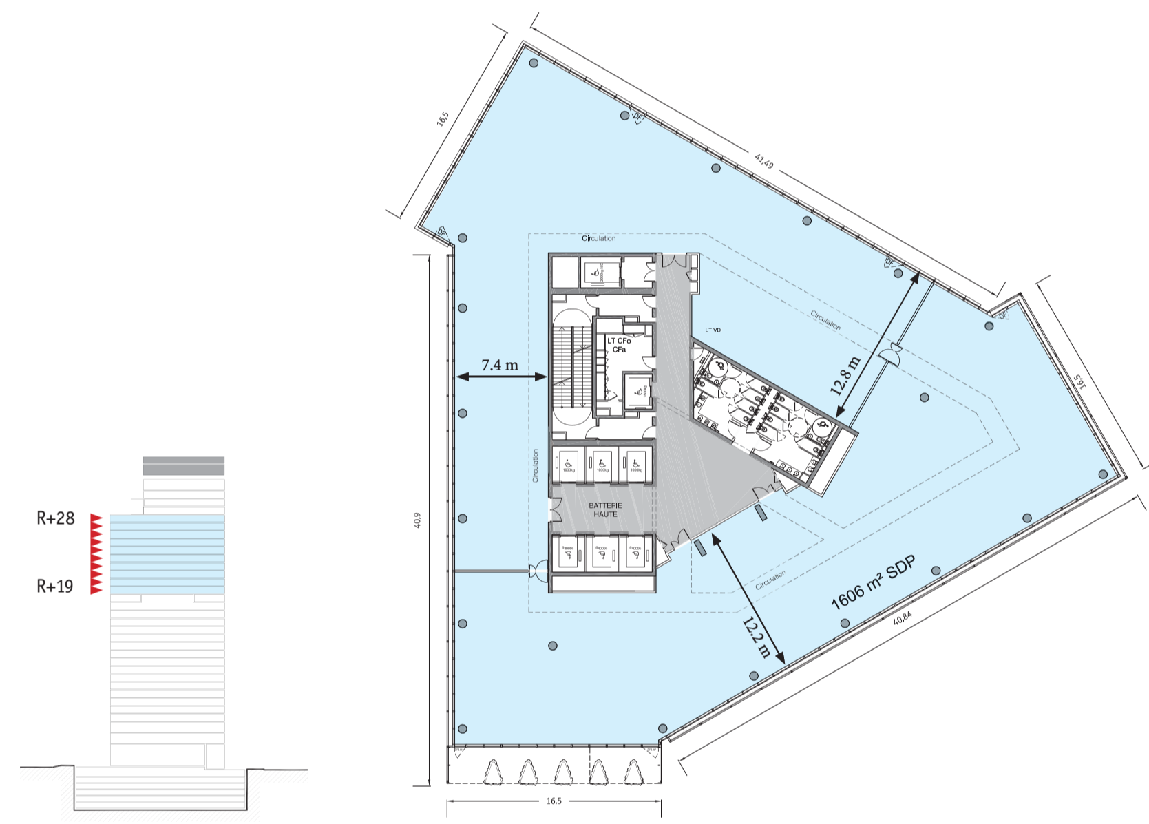
Plan type en batterie haute R+19 à R+28
