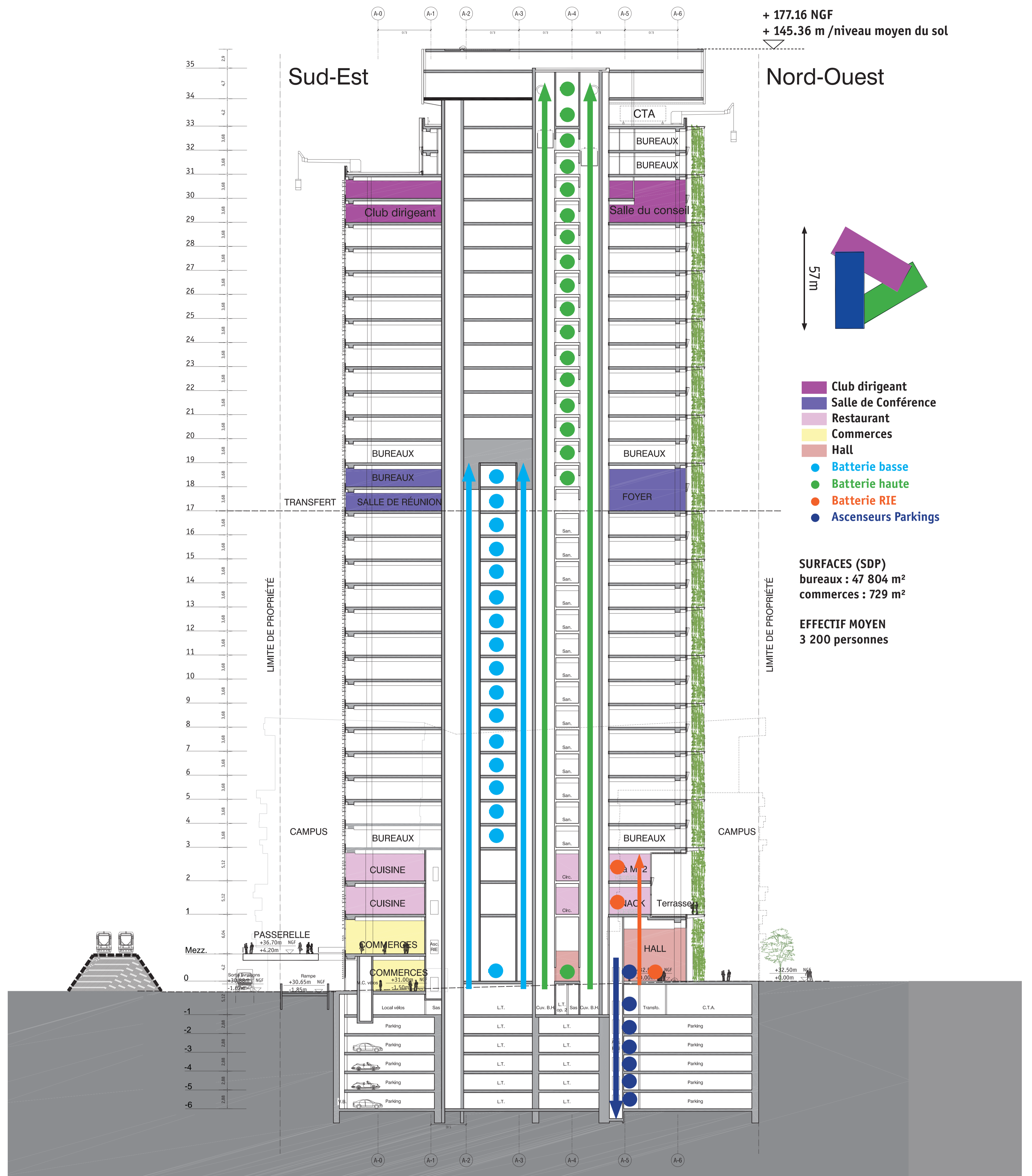
Coupe de principe de la tour
